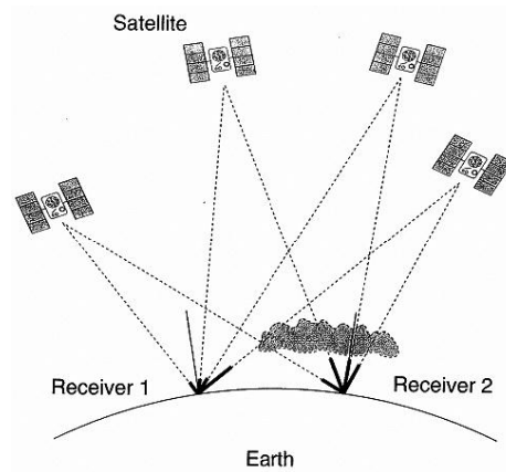
Satellitenvermessung (GPS), schematisch
