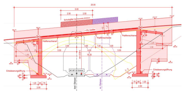
Projektierte Rahmenbrücke
