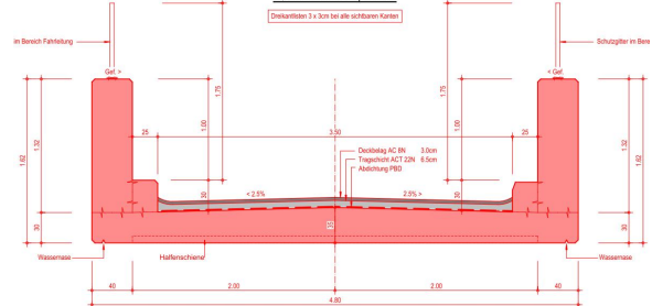
Querschnitt 1, 1: 20
